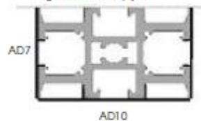
MSR afdeklijst voor BR75 / BR125
